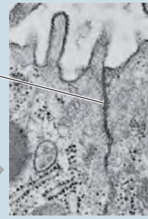
TEM 0.5 μm
