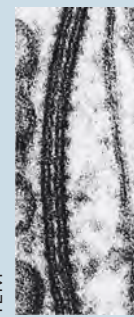
TEM 1 μm
