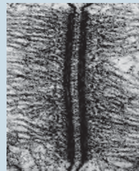
TEM 1 μm
